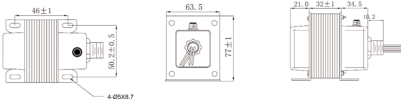
Type FMBAW1X
