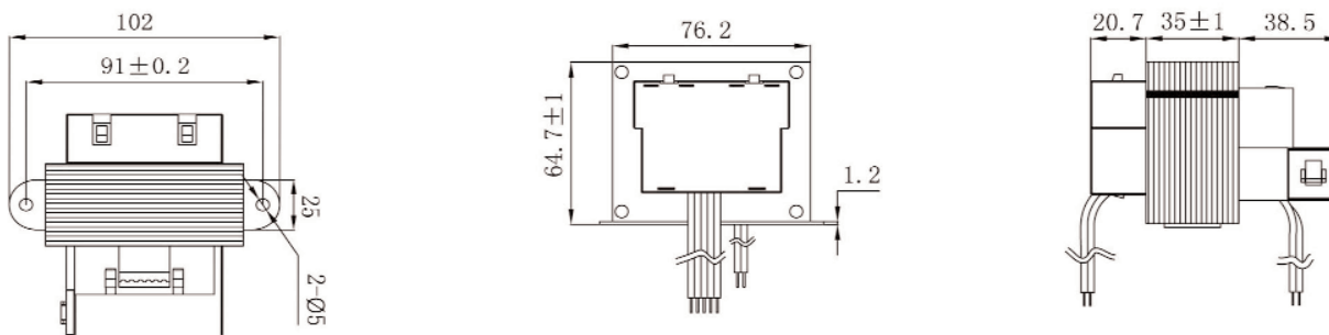
Type FMWX
